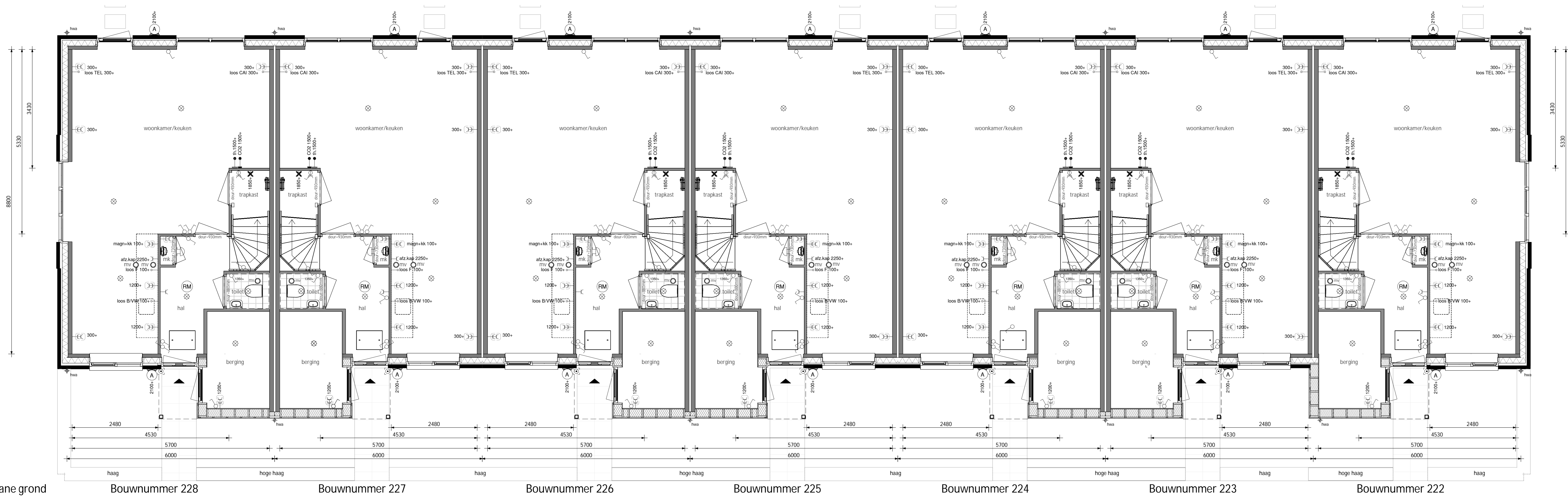
Begane grond Bouwnummer 228 Bouwnummer 227 Bouwnummer 226 Bouwnummer 225 Bouwnummer 224 Bouwnummer 223 Bouwnummer 222
