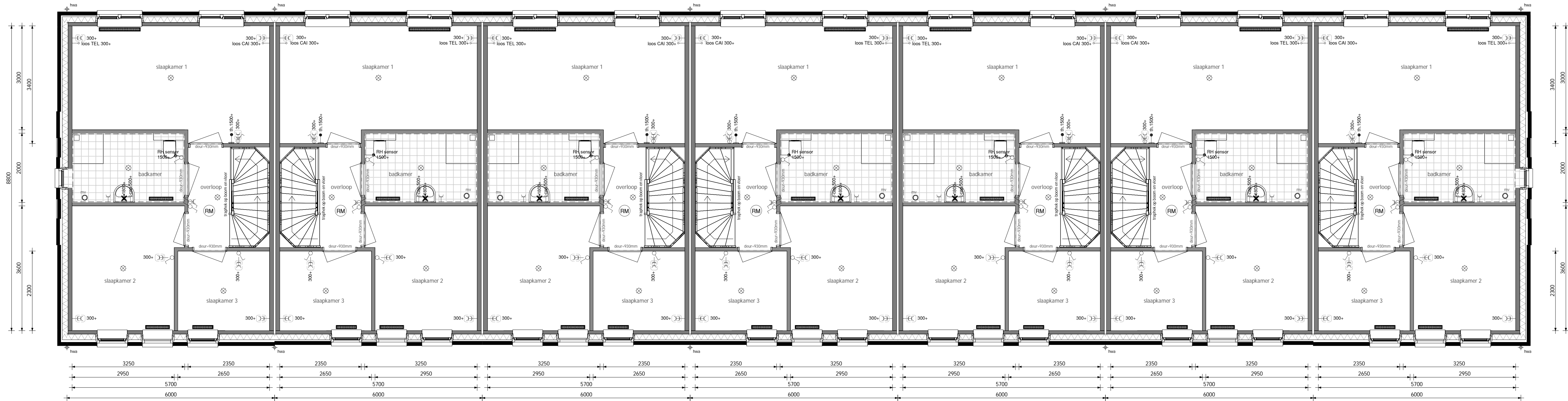
1e verdieping Bouwnummer 228 Bouwnummer 227 Bouwnummer 226 Bouwnummer 225 Bouwnummer 224 Bouwnummer 223 Bouwnummer 222
